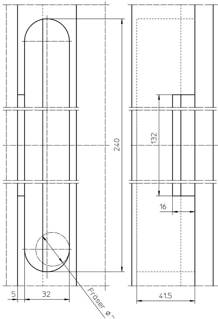
MILLING : FRAME
